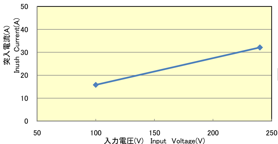
図4 突入電流特性(入力電圧に対して) Fig.4 Inrush Current Characteristics (vs Input Voltage)
