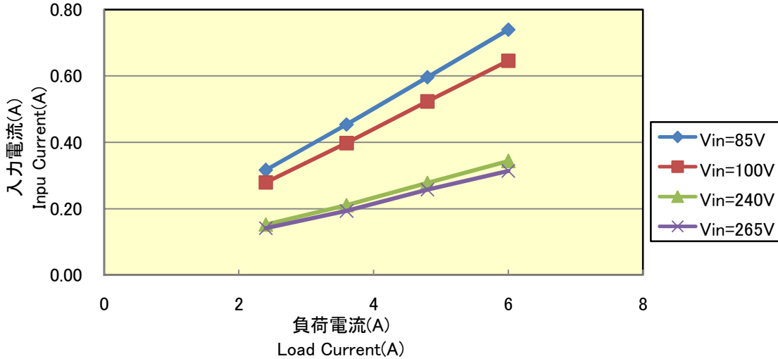
図1 入力電流特性(負荷電流に対して) Fig.1 Input Current Characteristics (vs Load Current)
