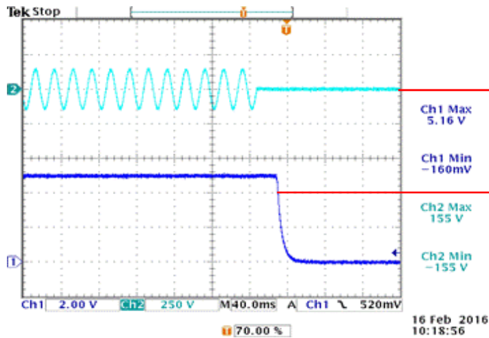
图16 出力電圧立下り波形 Fig.16 Output Voltage Falling Waveform
