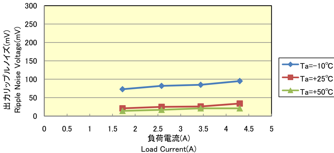
図9 リップルノイズ電圧特性(負荷電流に対して) Fig.9 Ripple Noise Voltage Characteristics (vs Load Current)
