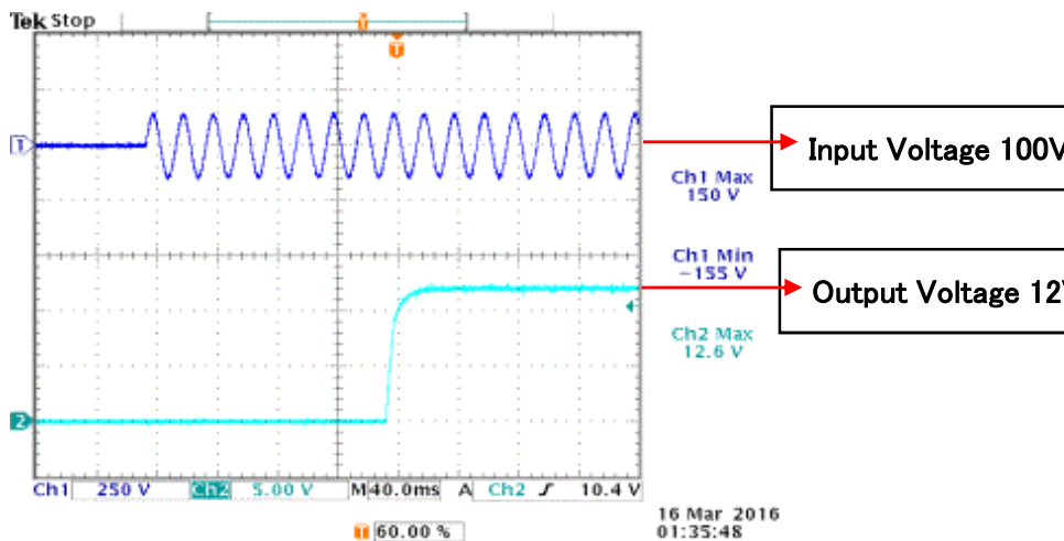
図15 出力電圧立上り波形 Fig.15 Output Voltage Rising Waveform
