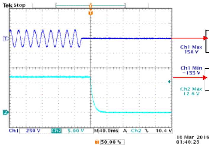
図16 出力電圧立下り波形 Fig.16 Output Voltage Falling Waveform
