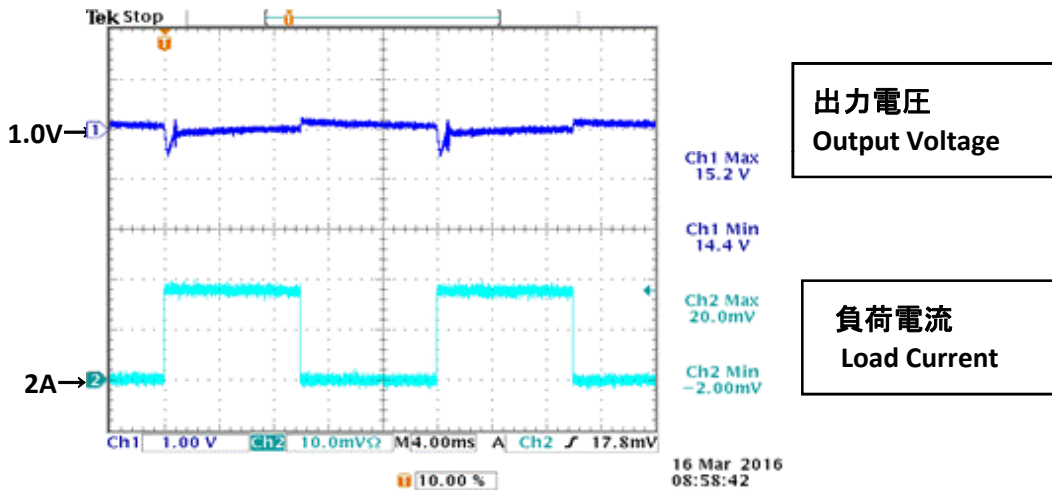
図14 ダイナミック時の負荷波形 Fig.14 Dynamic Load Waveform
