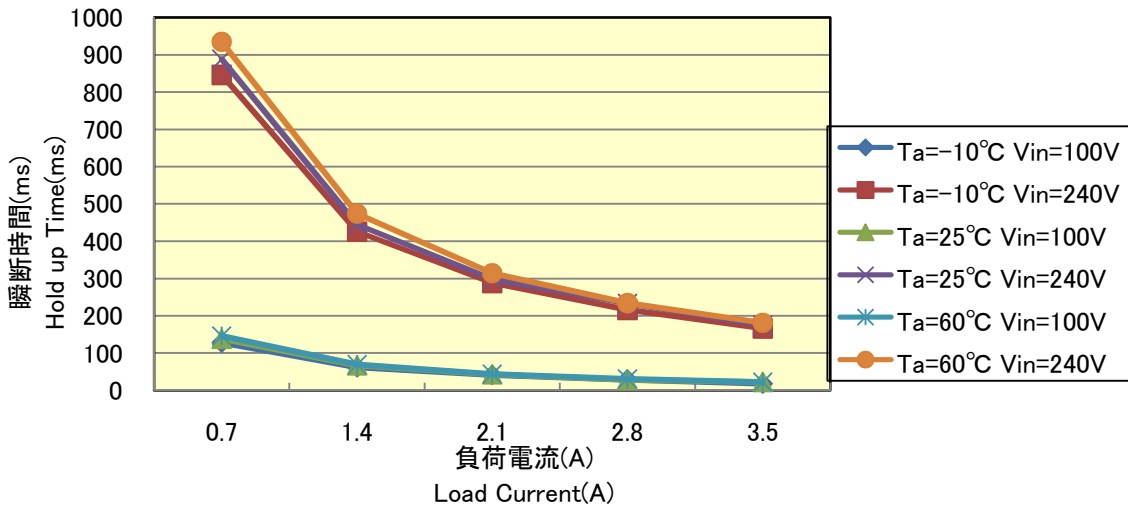
図13 入力瞬断時間(負荷電流に対して) Fig.13 Hold up time Characteristics (vs Load Current)
