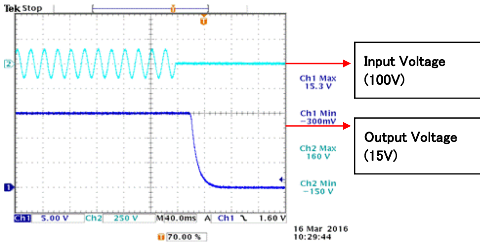
図16 出力電圧立下り波形 Fig.16 Output Voltage Falling Waveform
