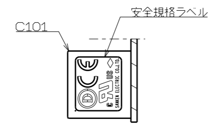
断面図 A-A (1:1)
