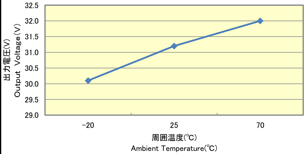
図7 過電圧特性(温度に対して) Fig.7 Over Voltage Protection Characteristics (vs. Temperature)
