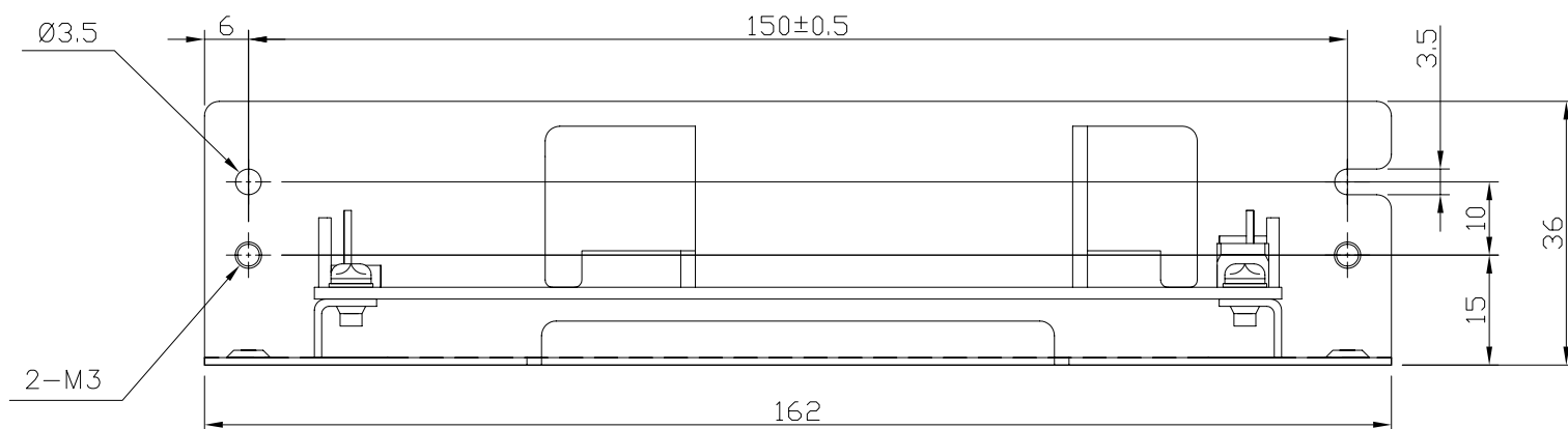
出力電圧可変ボリューム
