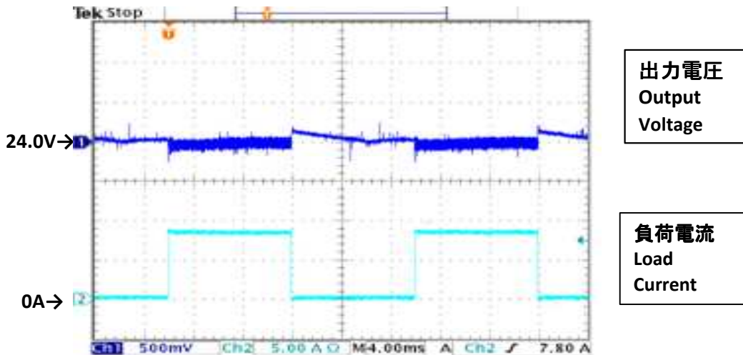
図14 タイミング時の負荷波形 Fig.14 Dynamic Load Waveform
