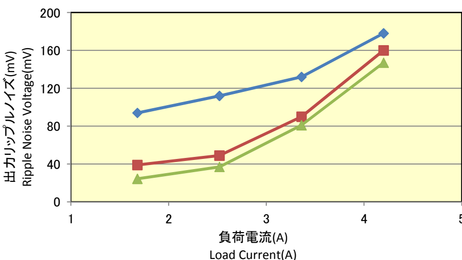
図9 リプルノイズ電圧特性(負荷電流に対して) Fig.9 Ripple Noise Voltage Characteristics (vs Load Current)
