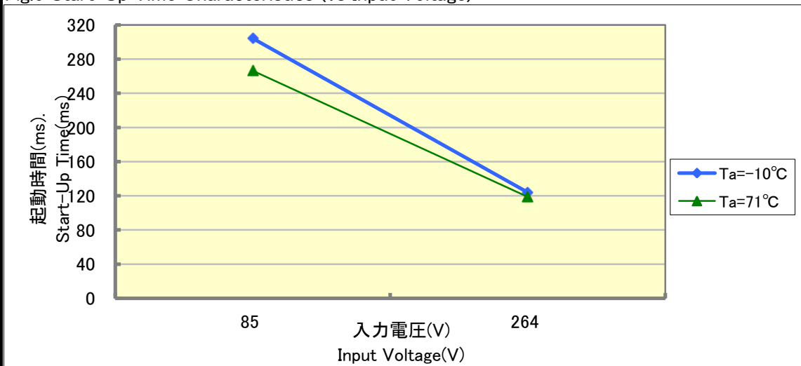
図5 起動時間特性(入力電圧に対して) Fig.5 Start-Up Time Characteristics (vs Input Voltage)
