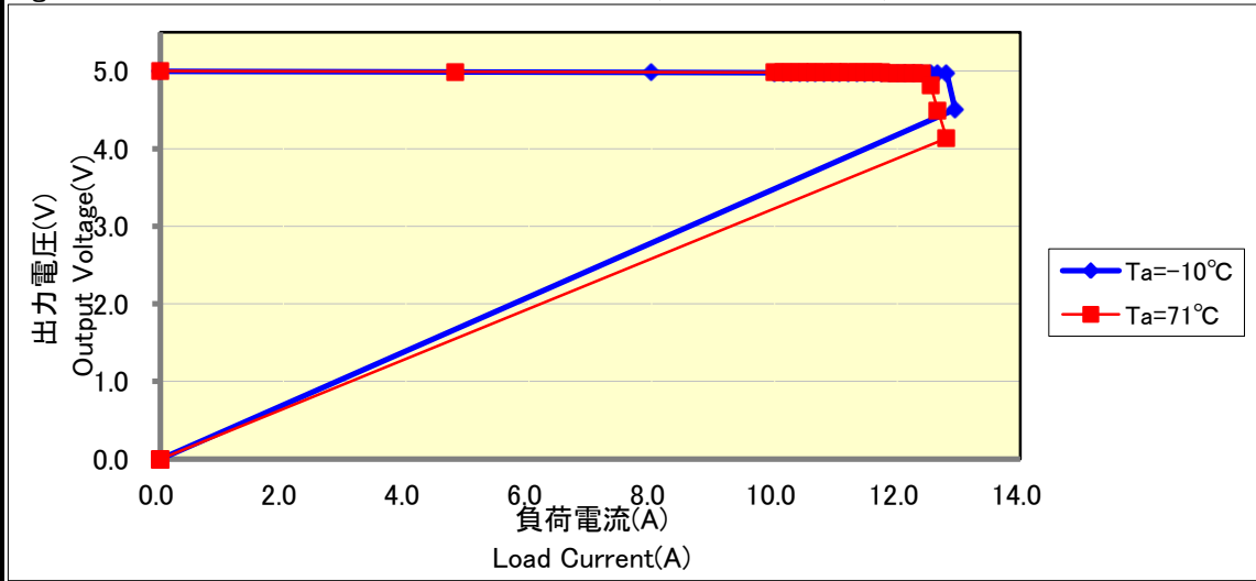
図10 過電流特性(負荷電流に対して) Fig.10 Over Current Protection Characteristics (vs Load Current)
