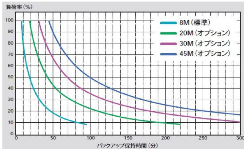
SFUシリーズ 負荷率とバックアップ時間 代表値 (参考値) 条件：初期特性，抵抗負荷，周囲温度 + 25℃
